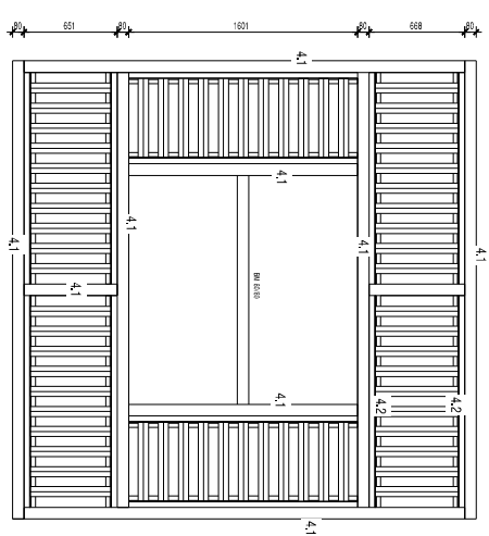
CADRE BOIS DEVANT SALLE DE REUNION 1/20
