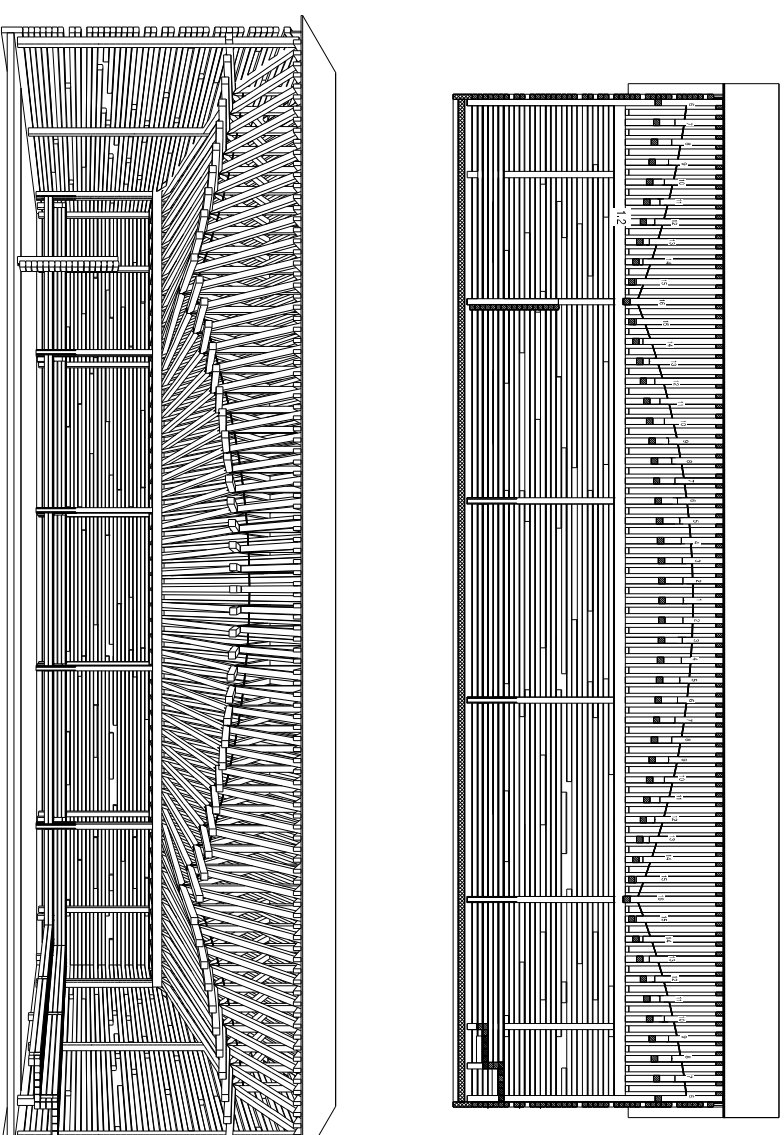
COUPE LONGITUDINALE 1/50
